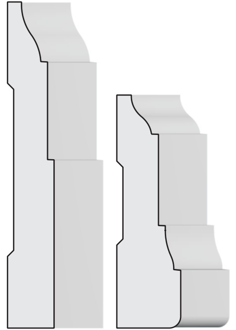
TS-BA 9 3 ½ X ½
