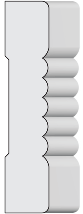
TS-CA 27 3 5/8 X 3/4
