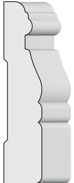
TS-CA 41 3 1/4 X 11/16
